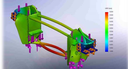
Simulación de esfuerzo de nuestros diseños
